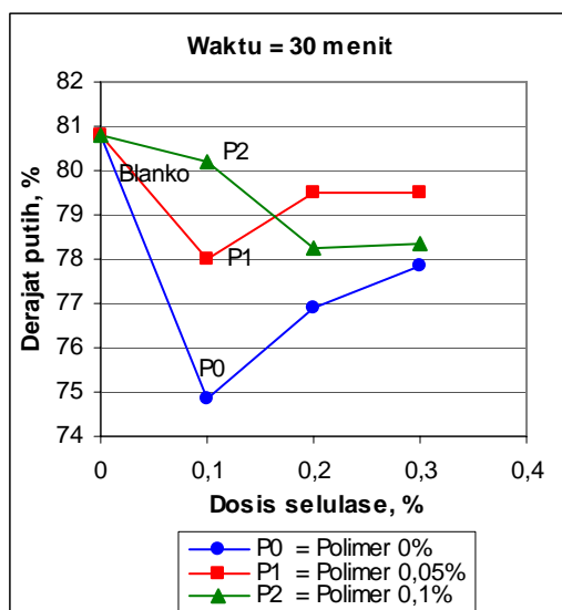
Gambar 6. Derajat Putih
