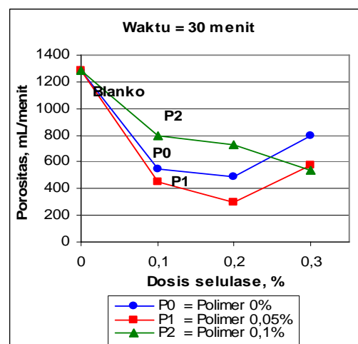
Gambar 5. Porositas
