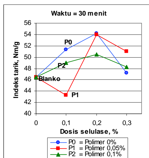
Gambar 2. Indeks Tarik
